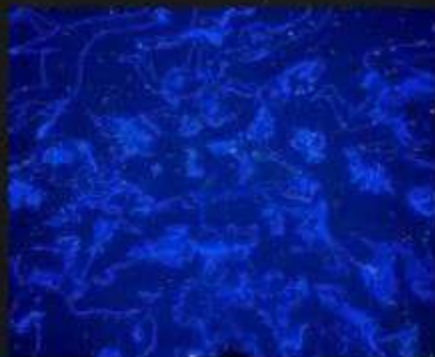
COSTELLAZIONI
